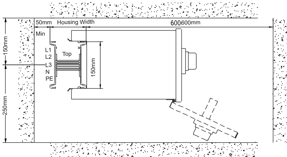
252A-500A插接箱安装所要求的空间
