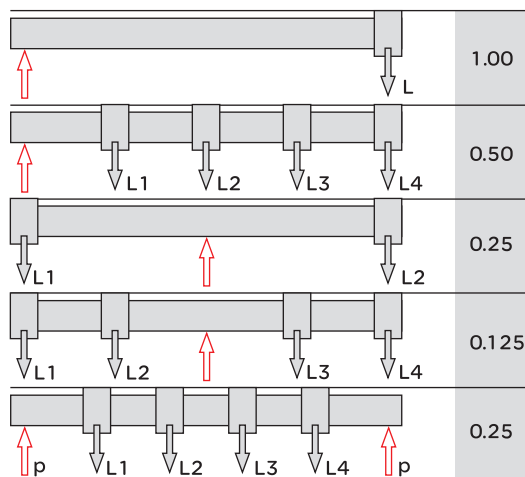
负载分布系数
