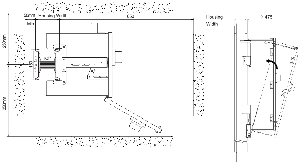
252A-500A插接箱安装所要求的空间
